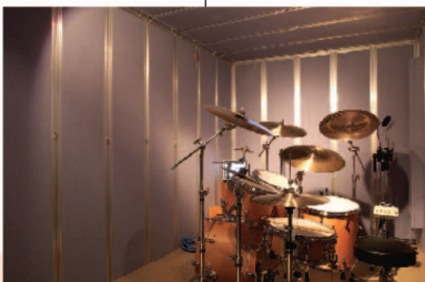
Recording Booth 遮音性能55dB、2層構造のメイン録音ブース、広さ約8畳。
